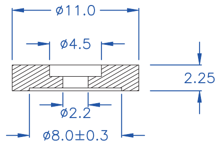
剖面圖:A-A
