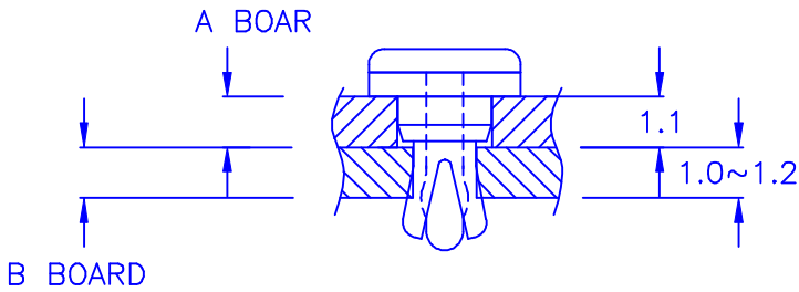
◎組裝示意圖
