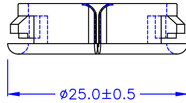
樣品裝置於 \phi 22.0 裝配孔量測
