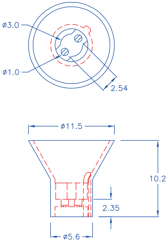
適用 \phi 3.0 \pm 0.25 (2PIN)LED燈
