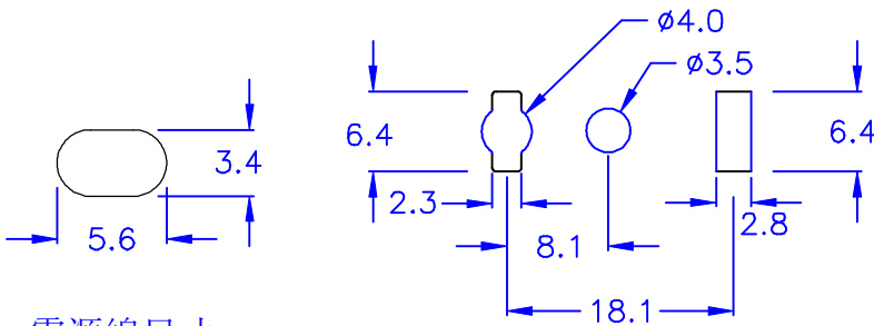
電源線尺寸
