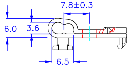
閉合示意圖
