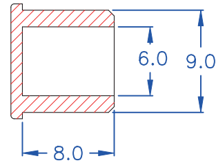
剖面圖 A-A
