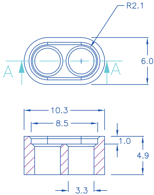
剖面圖 A-A
