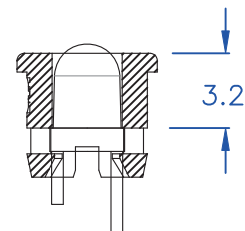
組裝示意圖
