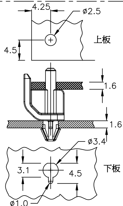
裝配孔示意圖
