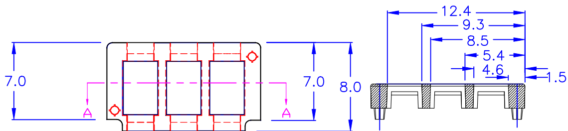
SECTION A-A
