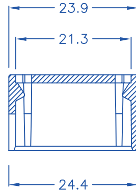
剖面圖A-A
