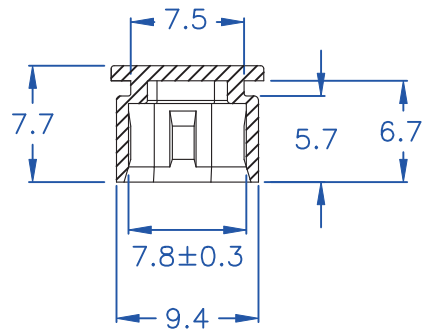
剖面圖 A-A
