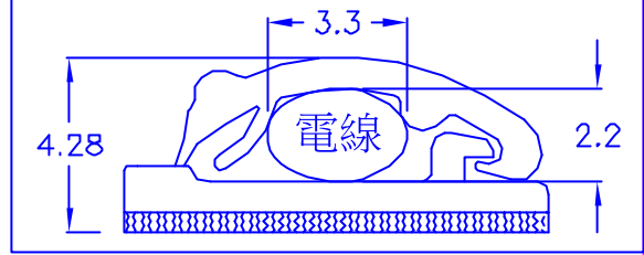
組裝示意圖
