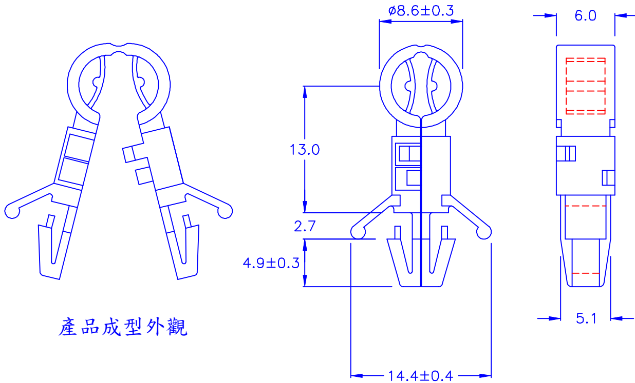
產品閉合尺寸圖
