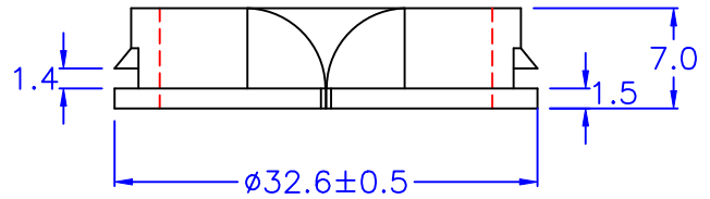
樣品裝置於 \phi 29.0 板厚 1.1mm 裝配孔量測
