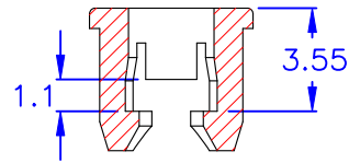
剖面圖 A-A
